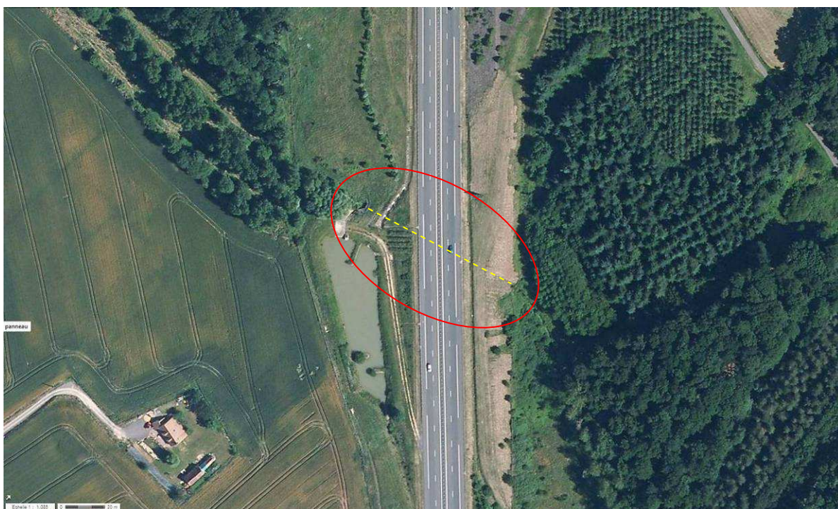
A28 Pr 122,4 - Buse de 85 m de longueur et 1,50 m de diamètre.
