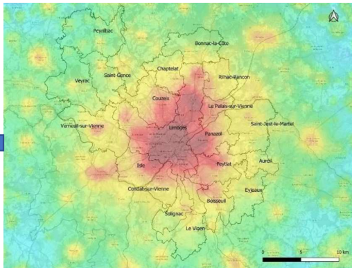
Simulation de la pollution lumineuse à partir de radiance satellite
