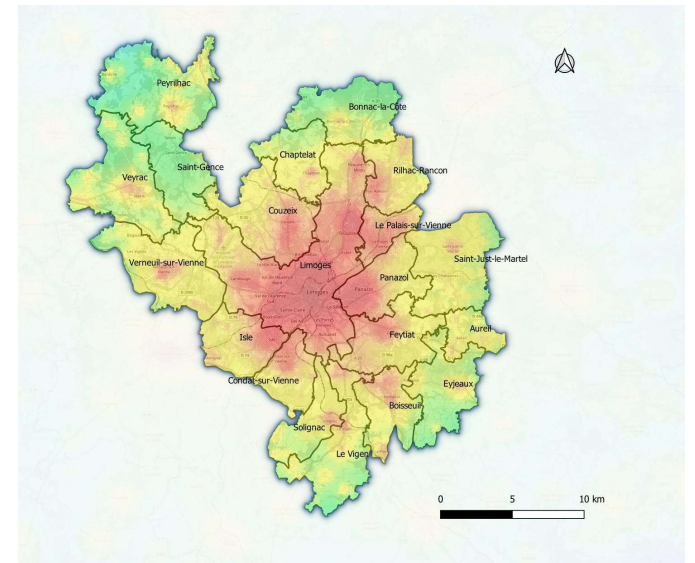
Modélisation de la pollution lumineuse
