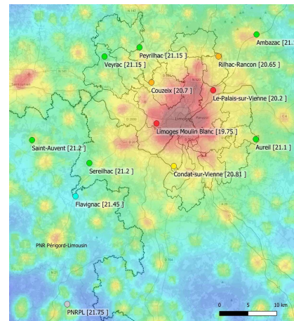
Mesures de la qualité du ciel sur le terrain (306 nuits, 13 sites)
